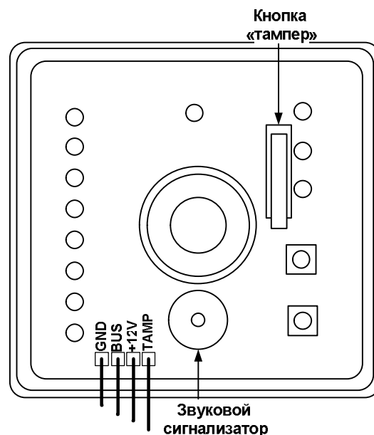
Рисунок 4 Индикатор зон «Линд – 7» со снятой крышкой
